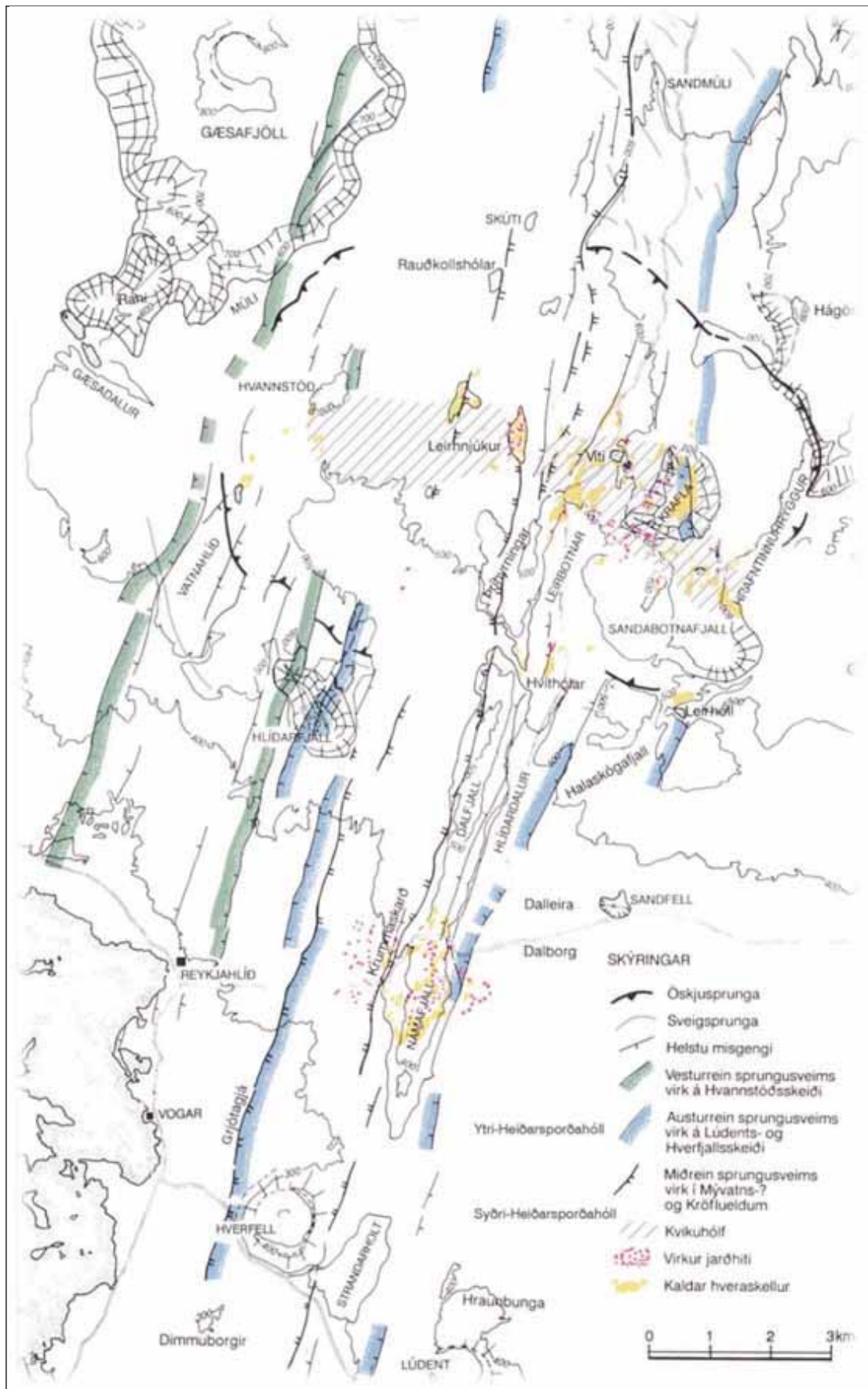
Mynd 2 Brotakerfi Kröflueiðstöðvarinnar (Kristján Sæmundsson, 1991).
